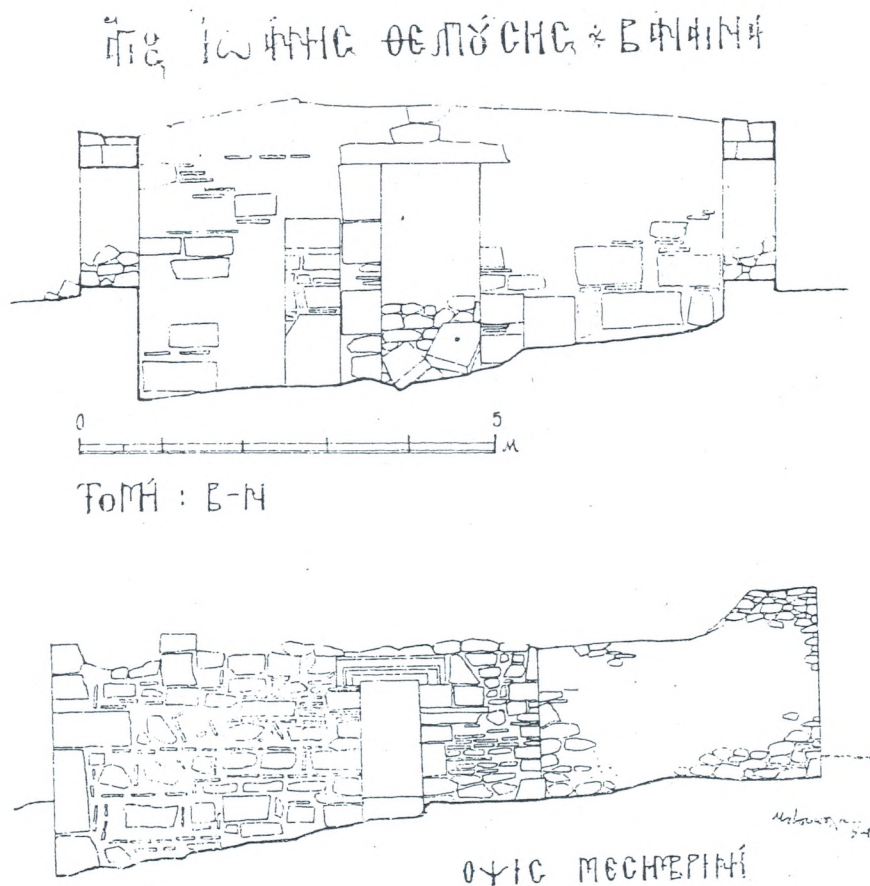
Εἰκ. 2. Ὁ Ἅγιος Ἰωάννης Θελπούσης. Τομή καὶ μεσημβρινή ὄψις.
