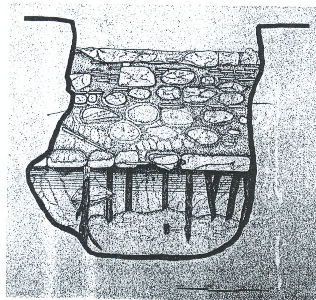
Σχ. 3. Τομή τμήματος του περιτειχίσματος με τη θεμελίωση και την πασσαλόπληξη.
