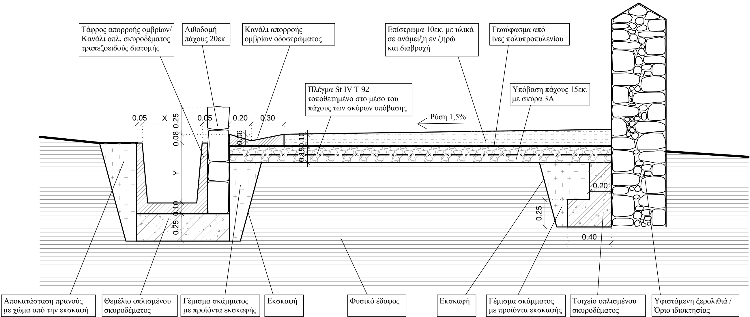
ΤΥΠΙΚΗ ΤΟΜΗ ΜΟΝΟΠΑΤΙΟΥ ΣΕ ΕΠΑΦΗ ΜΕ ΥΦΙΣΤΑΜΕΝΗ ΛΙΘΟΔΟΜΗ
