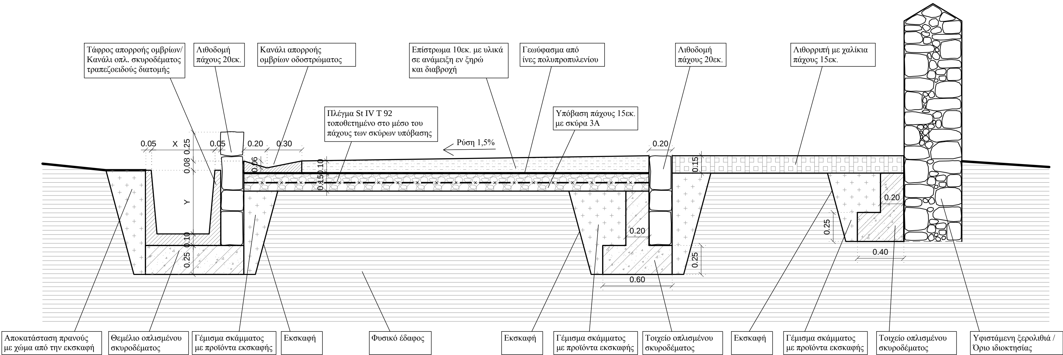
ΤΥΠΙΚΗ ΤΟΜΗ ΜΟΝΟΠΑΤΙΟΥ ΠΕΡΙΟΧΗ ΜΕ ΟΔΟΣΤΡΩΜΑ ΚΑΙ ΜΗ ΒΑΤΗ ΖΩΝΗ
