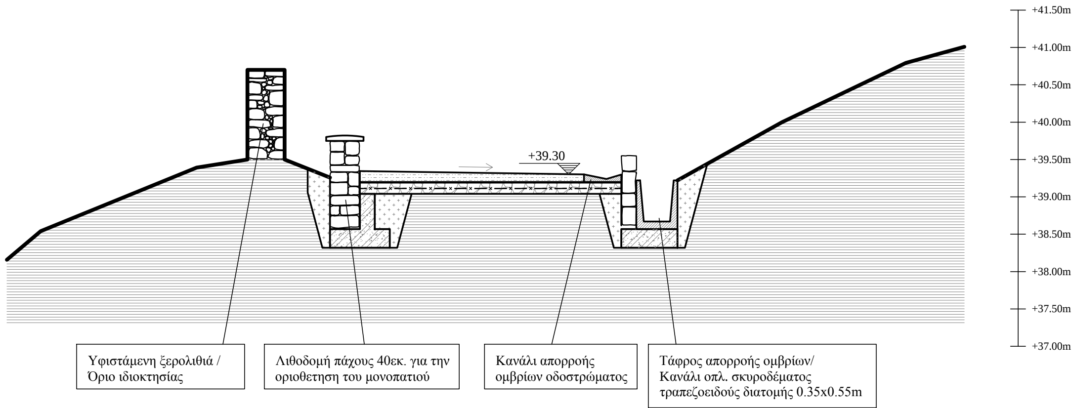
ΤΟΜΗ Κ-Κ
