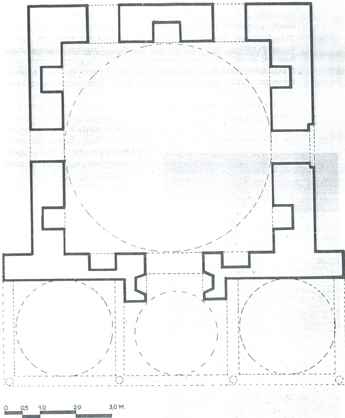
Σχέδ. 1. Κάτοψη τού τάφου
