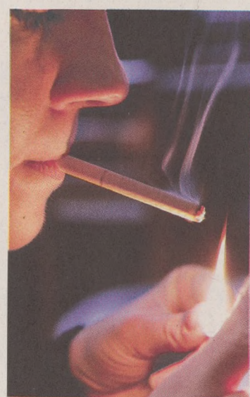
Το πολώνιο-210 είναι ο ένοχος μόλυνσης του φυτού του καπνού.
