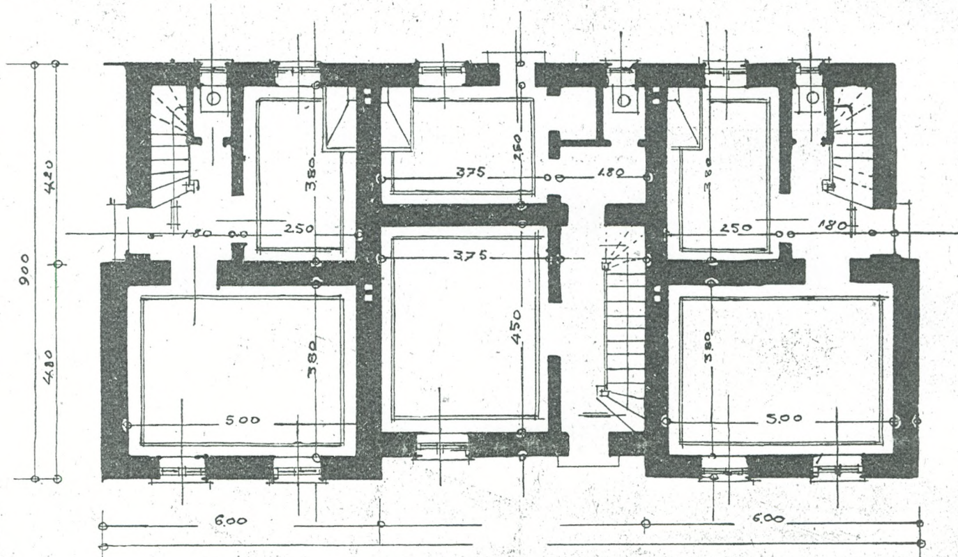
Εἰκ. 7.— Κάτωφιν ἰσογείου συγκροτήματος, οἰκημάτων τύπου Θ συνοικισμοῦ Βύρωνος.—Κλίμαξ 1:100.
