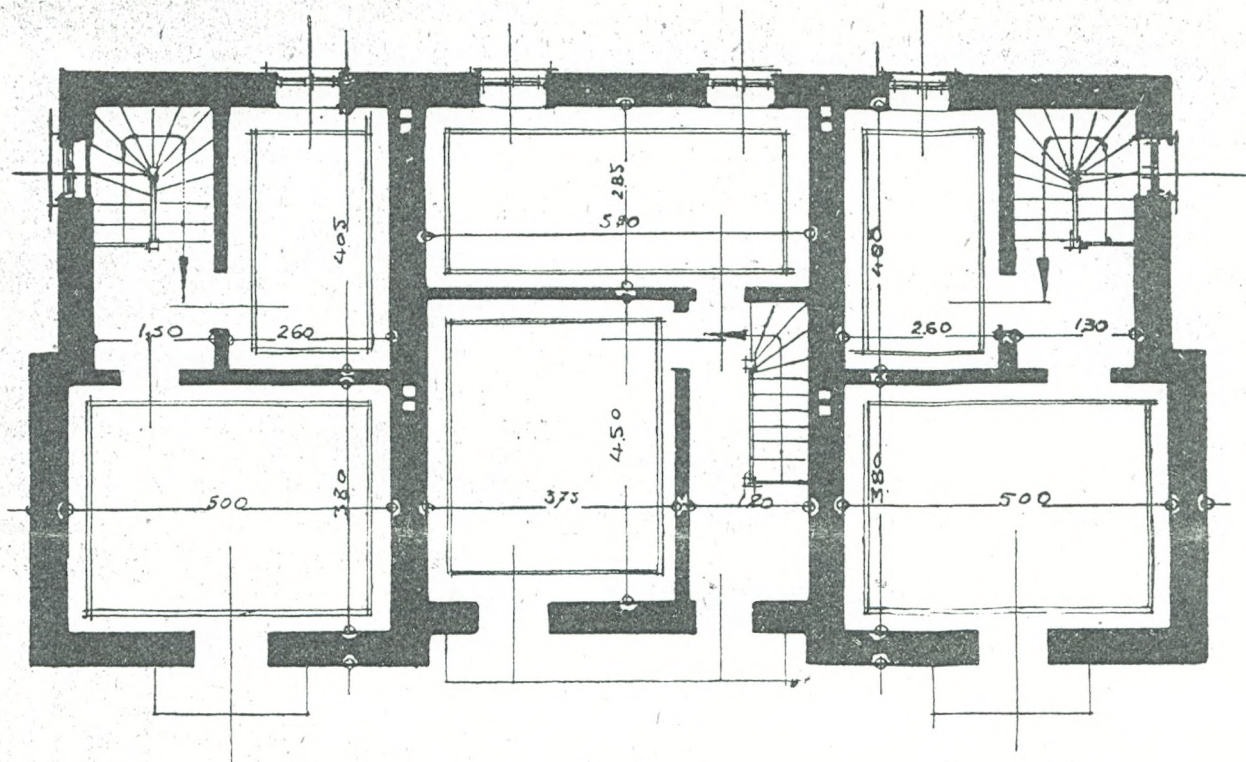
Εἰκ. 6.—Κάτοπις ὁρόφου συγκροτήματος μονοκατοικιῶν συνοικισμοῦ Βύρωνος τύπου Θ—Κλίμαξ 1:100.
