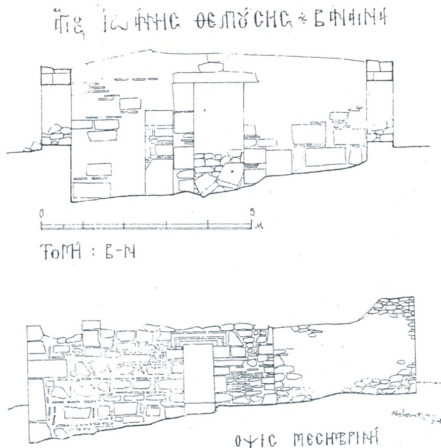
Εἰκ. 2. Ὁ Ἅγιος Ἰωάννης Θελπούσης. Τομή καὶ μεσημβρινὴ ὄψις.
