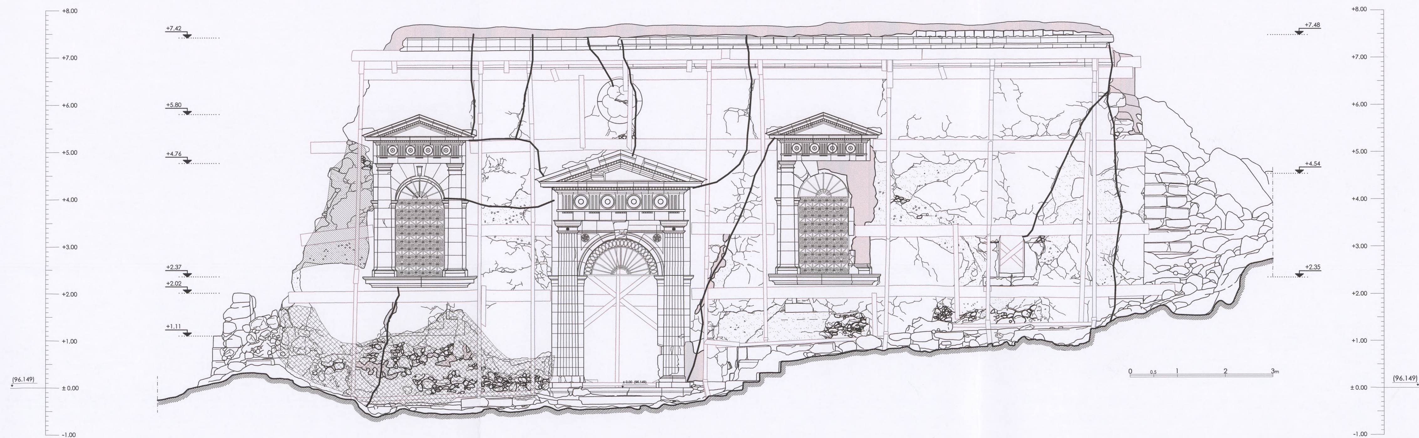
ΝΟΤΙΟΑΝΑΤΟΛΙΚΗ ΟΨΗ
