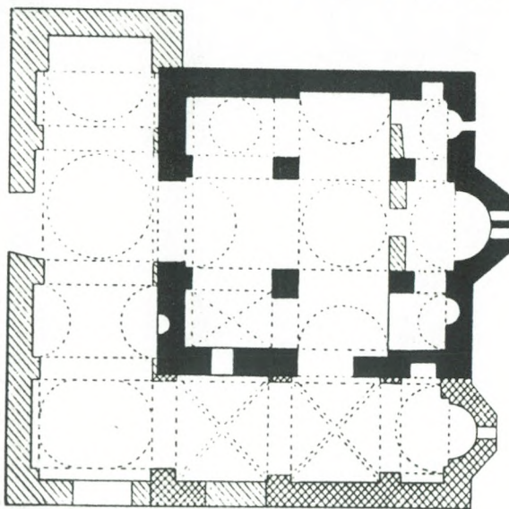
Είκ. 80. "Αθήνα, "Θορρη Εκκλησία, γ' τέταρτου 12ου αϊ. (κάτοψη).
