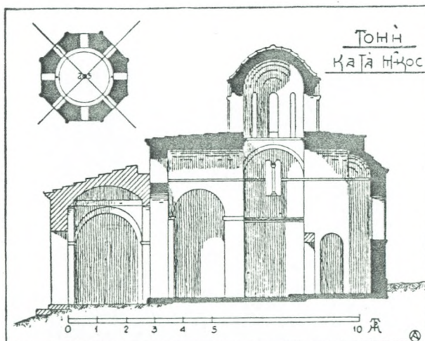
Εἰκ. 173. Τομὴ Ὁμορφης Ἐκκλησιᾶς.
