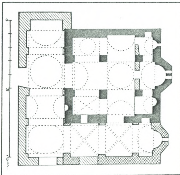
Εἰκ. 174. Κάτοπις Ὁμορφης Ἐκκλησιᾶς.
