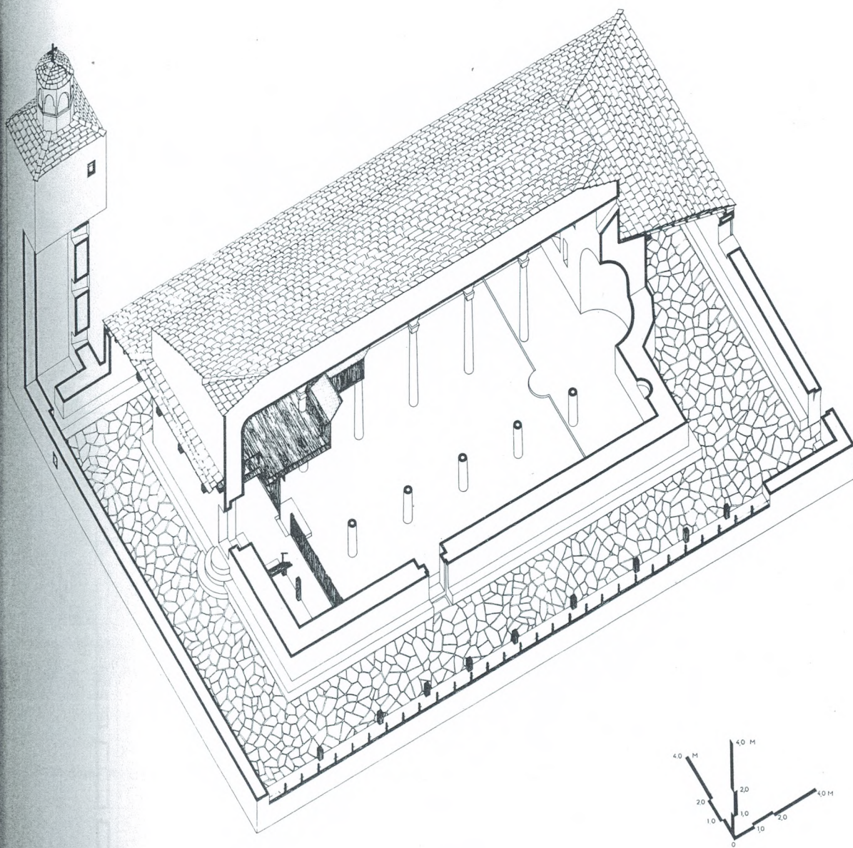
Ἀετοχώρι. Ἅγιος Δημήτριος (16). Ἀξονομετρικὴ τομὴ.
