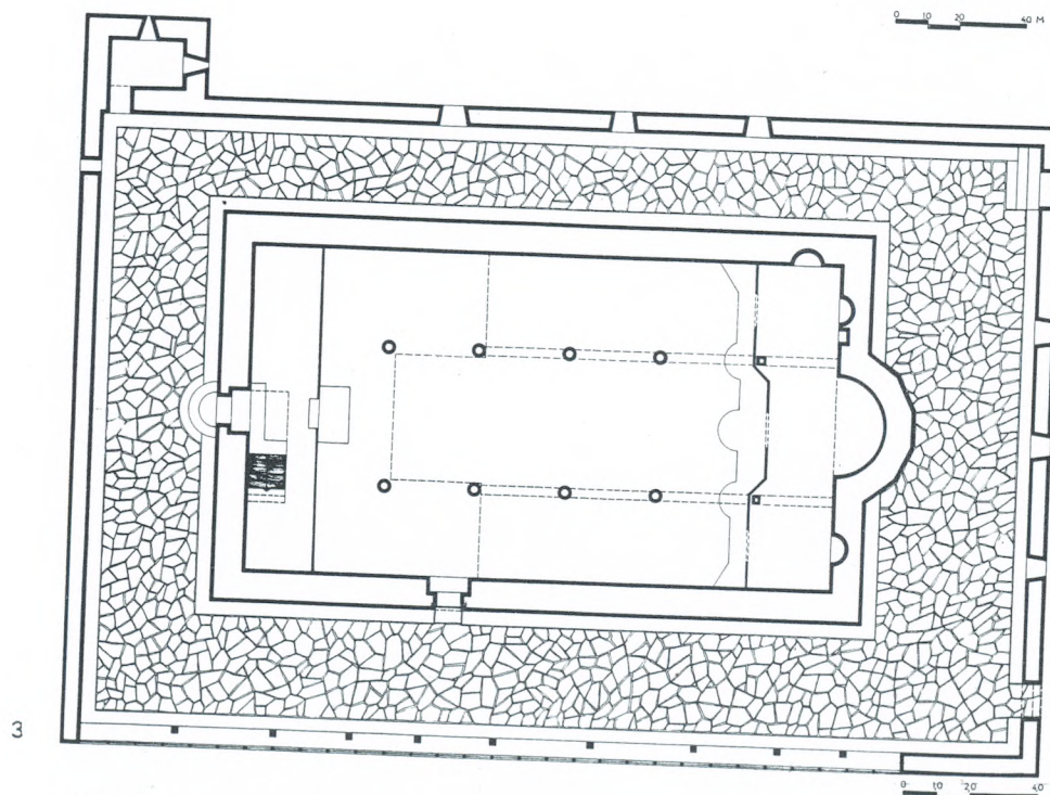
Ἄετοχώρι. Ἅγιος Δημήτριος (16). 1. Μεσημβρινή ὄψη. 2. Τομή κατὰ μῆκος. 3. Κάτοψη.
