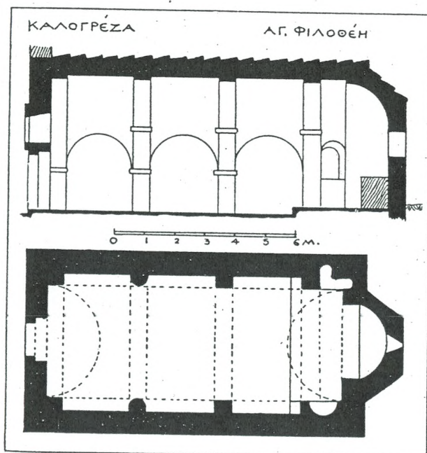
Εἰκ. 176. Κάτοψις καὶ τομή Ἀγ. Φιλοθέης.
