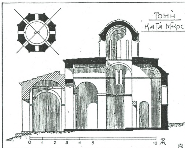
Εἰκ. 173. Τομὴ Ὁμορφης Ἐκκλησιᾶς.
