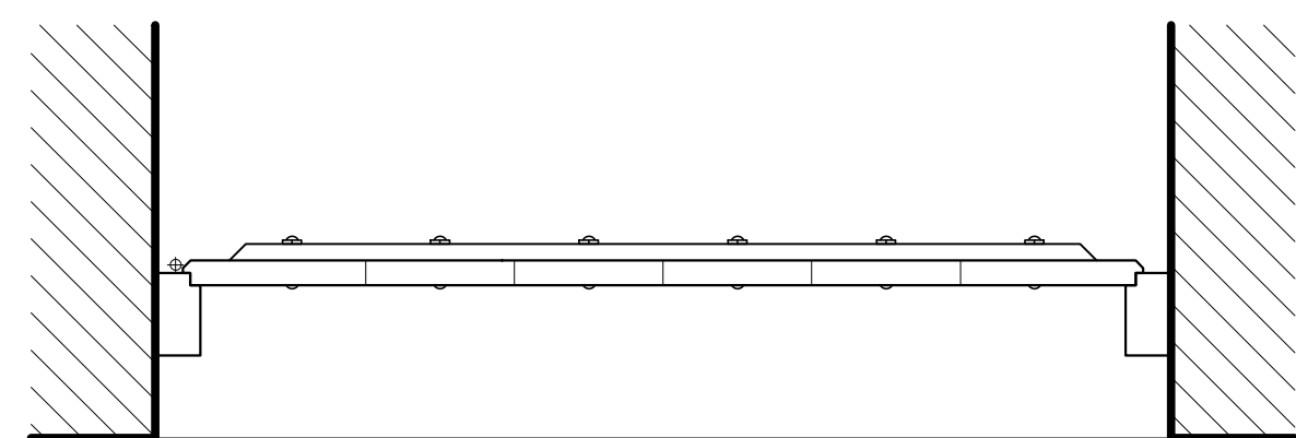
ΚΑΤΟΨΗ ΚΛΙΜΑΚΑ 1:10
