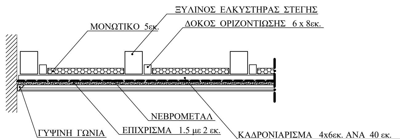
ΤΟΜΗ Β-Β ΚΛ. 1:10
