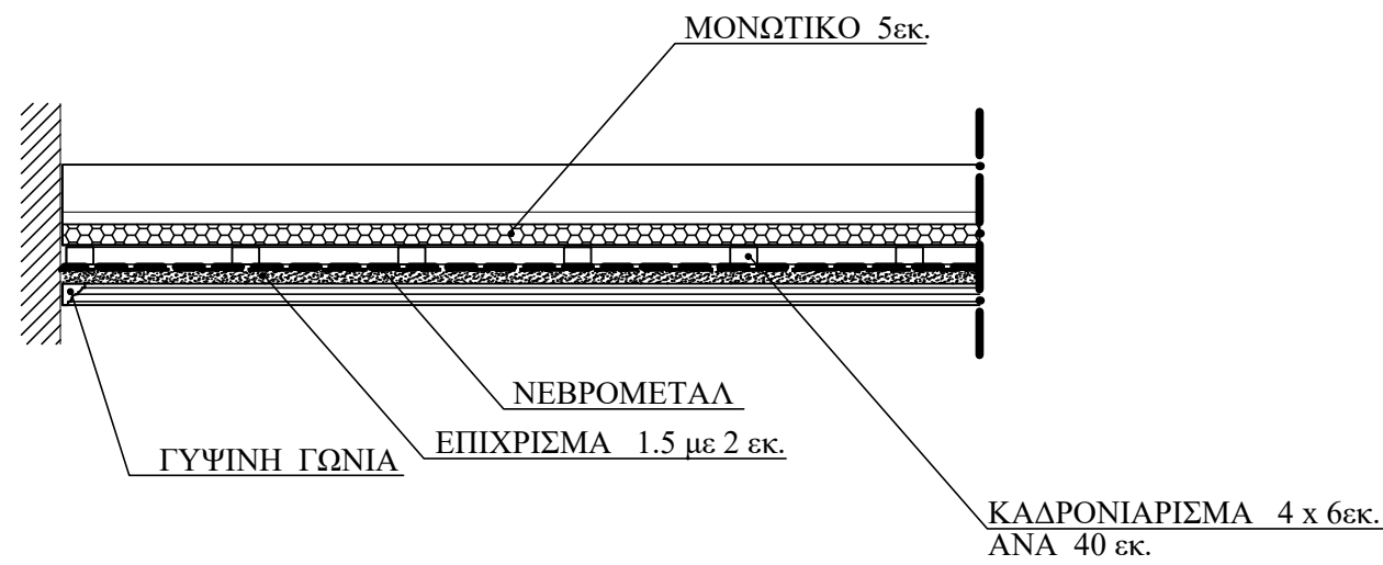
ΤΟΜΗ Α-Α ΚΛ. 1:10
