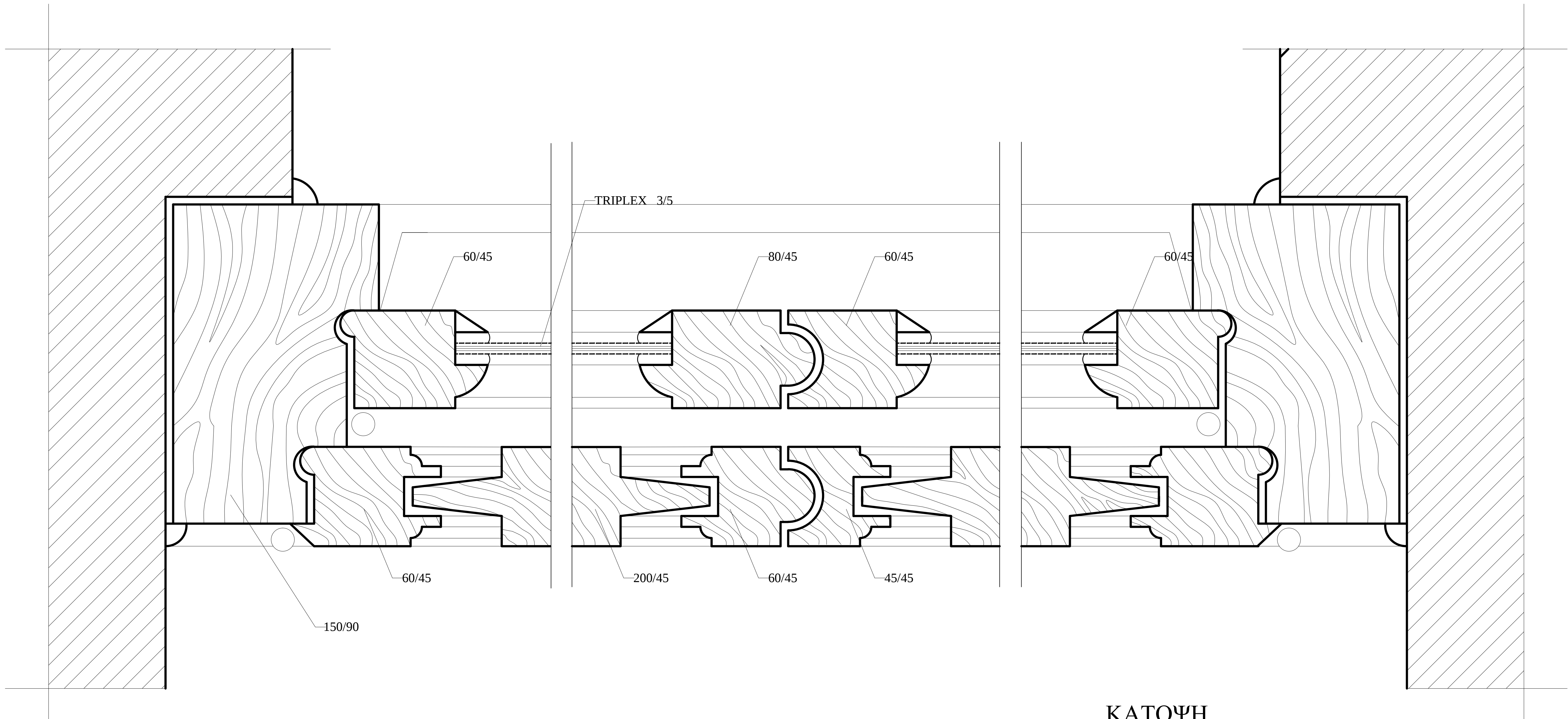
ΚΑΤΟΨΗ ΚΛΙΜΑΚΑ 1 : 1
