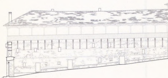
Νότια Όψη από την πρόταση για την αποκατάσταση της Βόρειας Πτέρυγας
