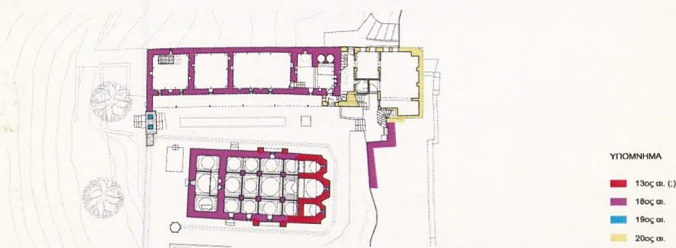
Κάτοψη της δεύτερης στάθμης του μοναστηριακού συγκροτήματος με τις οικοδομικές φάσεις
