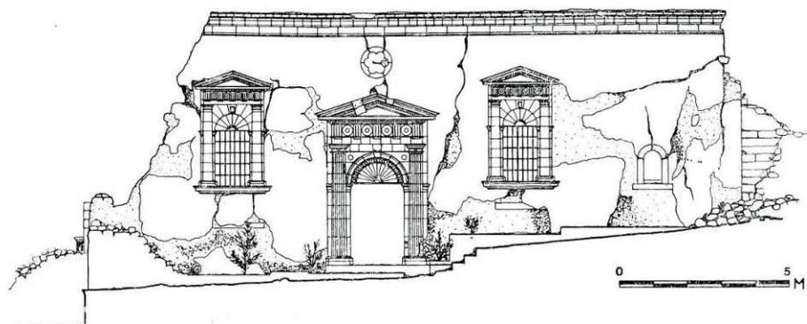
Εικ. 8. ΝΑ.. όψη του καθολικού της Μονής Σισίων, σχέδιο αποτύπωσης (Μπιρμπίλη 1991: 208, εικ. 12).
