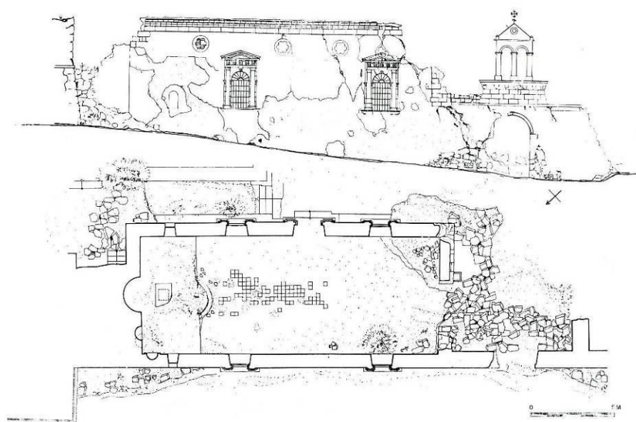
Εικ. 9. ΒΔ. όψη του καθολικού της Μονής Σισίων (άνω) και κάτοψη (κάτω), σχέδια αποτύπωσης (Μπιρμπίλη 1991:204, εικ. 3).
