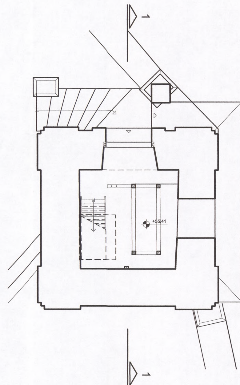
ΚΑΤΟΨΗ Β' ΣΤΑΘΜΗΣ
