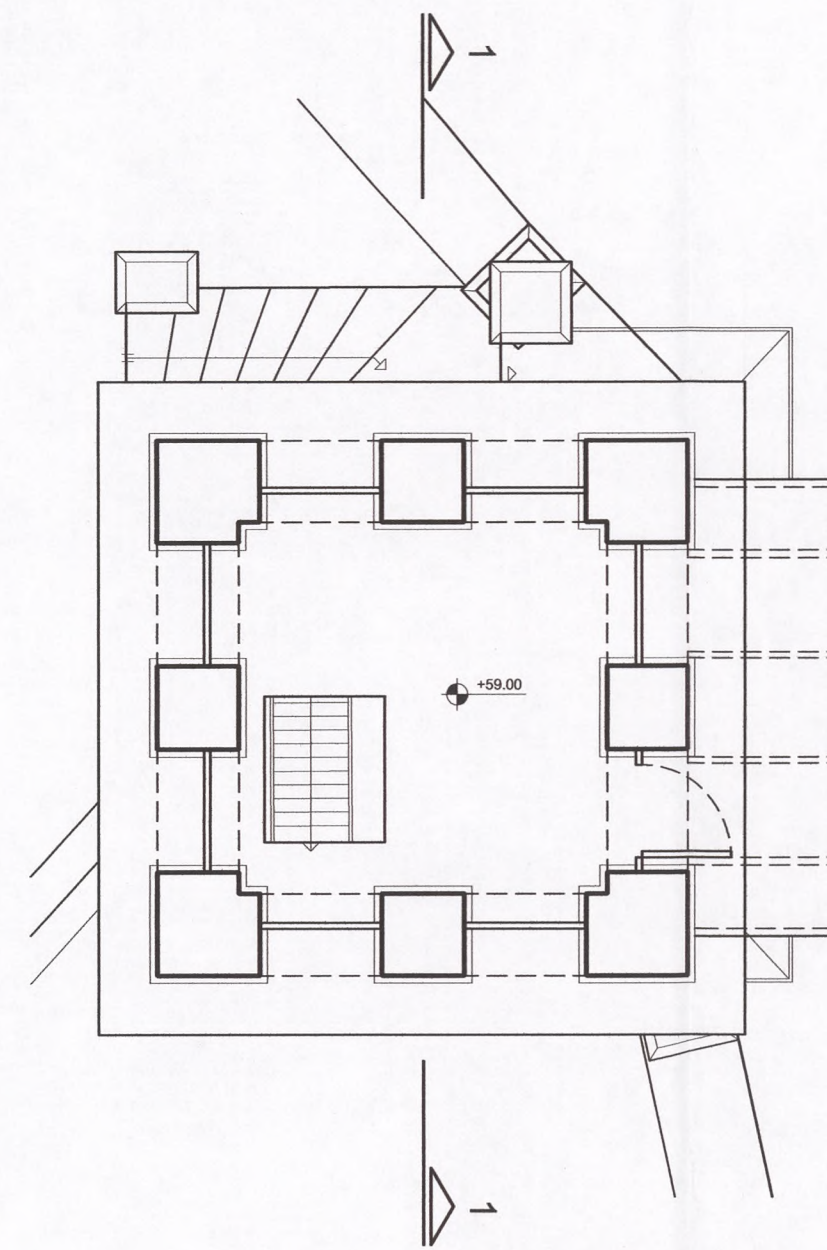
ΚΑΤΟΨΗ Γ' ΣΤΑΘΜΗΣ
