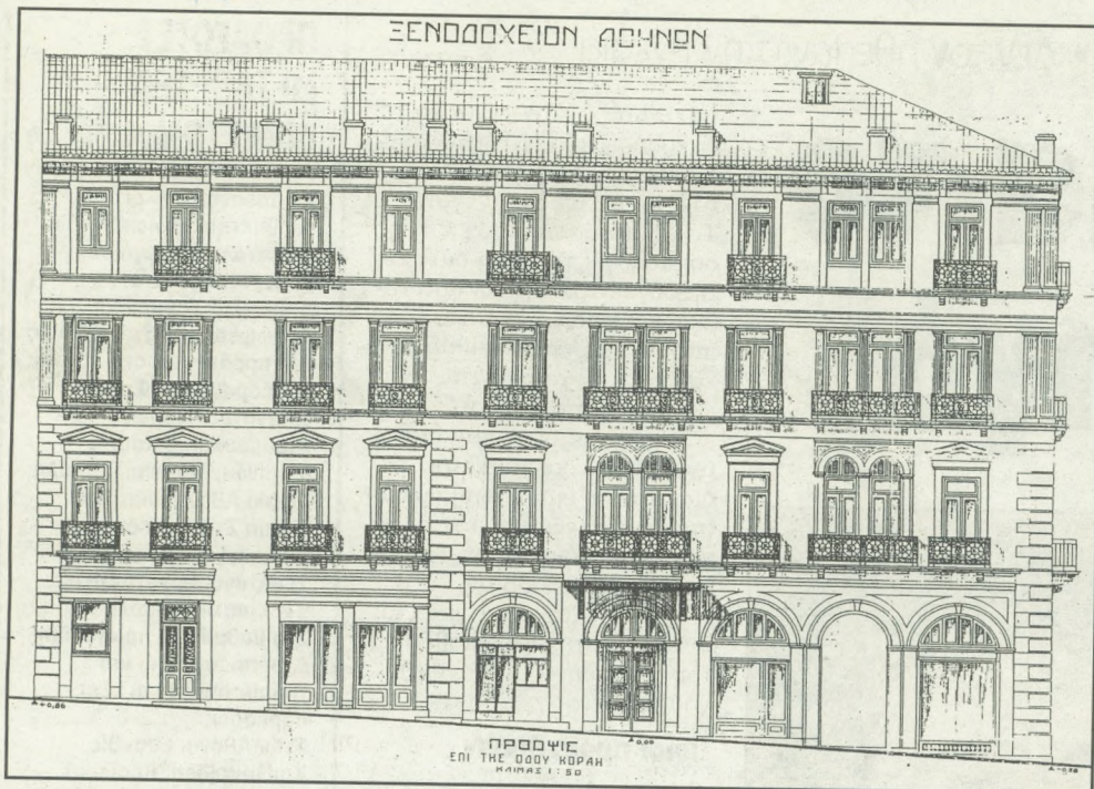
Η όψη του κτιρίου του Ξενοδοχείου Αθηνών (Σταδίου και Κοραή) το 1930, σε σχέδια του Ι. Αντωνιάδη. Προστέθηκε όροφος, αλλά σε απόλυτη μορφολογική και λειτουργική αντιστοιχία με το υφιστάμενο κτίριο
