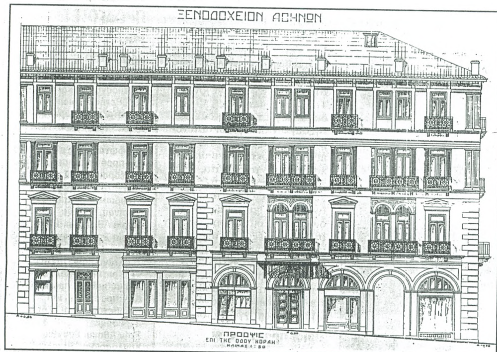
Η όψη του κυρίου του Ξενοδοχείου Αθηνών (Σταδίου και Κοραή) το 1930, σε σχέδια του Ι. Αντωνιάδη. Προστέθηκε όροφος, αλλά σε απόλυτη μορφολογική και λειτουργική αντιστοιχία με το υφιστάμενο κτίριο
