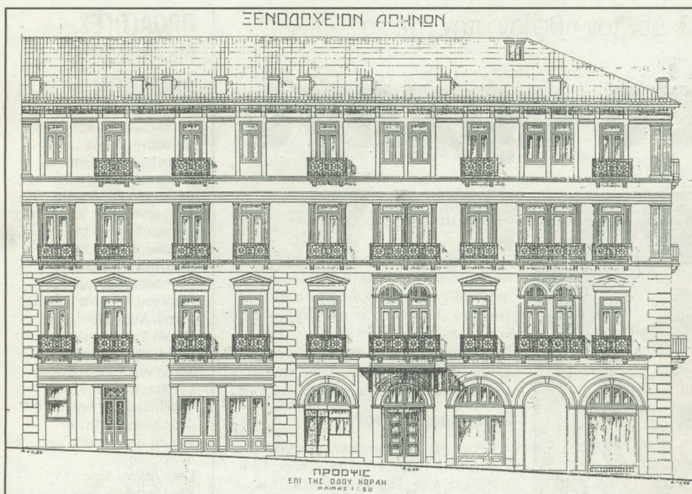
Η όψη του καρίου του Ξενοδοχείου Αθηνών (Σταδίου και Κοραή) το 1930, σε σχέδια του Ι. Αντωνιάδη. Προστέθηκε όροφος, αλλά σε απόλυτη μορφολογική και λειτουργική αντιστοιχία με το υφιστάμενο κτίριο
