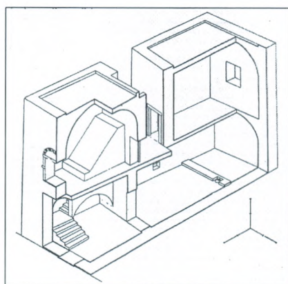
Αξονομετρική τομή οικίας στα Μεστά, Μιχελής.
