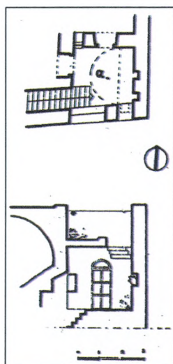
Κάτοψη και τομή ηλιακού σε οικία στο Πυργί, Μιχελής.
