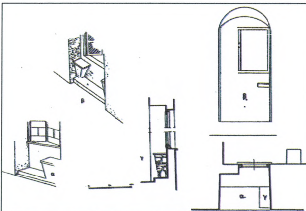
Εναλλακτικοί τρόποι εκμετάλλευσης του πλάτους του τοίχου στην ποδιά του παραθύρου, Μιχελής.
