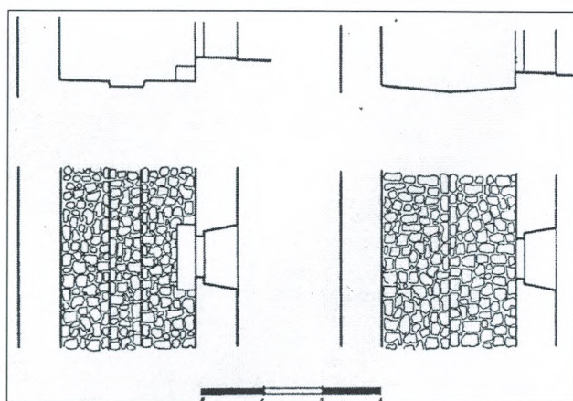
Τομές, κατόψεις δρόμων στα Μεστά και στην Καλαμωτή, Μιχελής.
