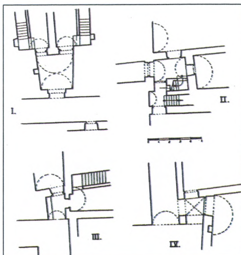
Περιπτώσεις διάταξης της εισόδου, Μιχελής.
