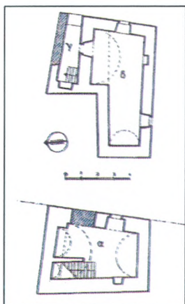
Κατόψεις όλων των επιπέδων μονόχωρης οικίας, Μιχελής.
