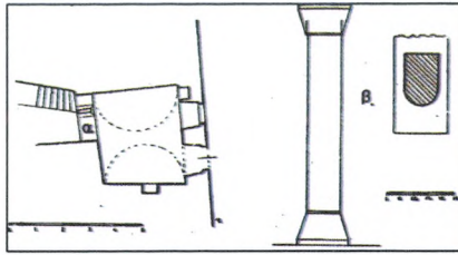
Ο «μπαλός», κάτοψη εισόδου και λεπτομέρεια κίονα, Μιχελής.
