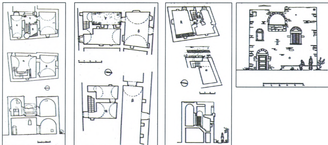
Οικίες με ανοικτό ηλιακό, κλειστό ηλιακό και ηλιακό σε δύο επίπεδα αντίστοιχα, Μιχελής.
