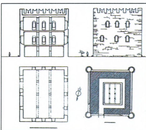
Αναπαράσταση κεντρικού πύργου Πυργίου και γενικού διαγράμματος οχυρώματος, Μιχελής.
