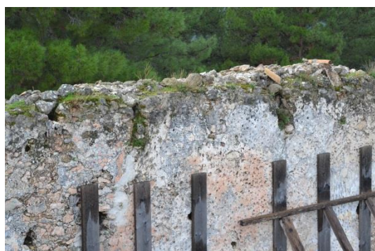
Εικ. 60 Η απόληξη του νότιου τοίχου από το εσωτερικό.
