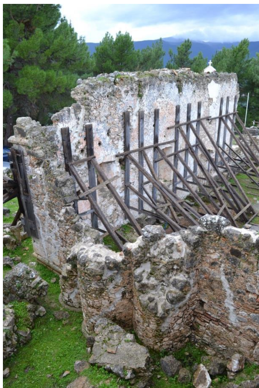
Εικ. 51 Άποψη του καθολικού από τον πύργο.
