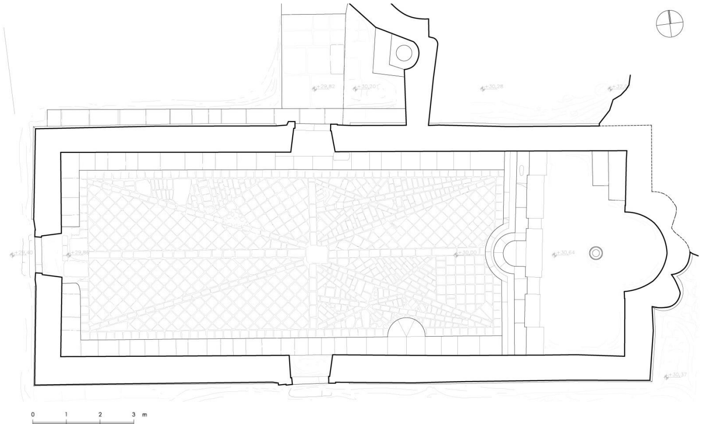
Εικ. 13 Κάτοψη του καθολικού.
