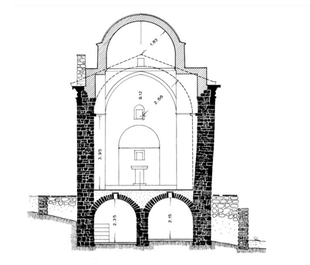
Εγκάρσια τομή 4-4 | κλίμακα 1:200
