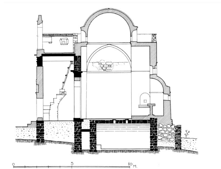
Κατά μήκος τομή 1-1 | κλίμακα 1:200
