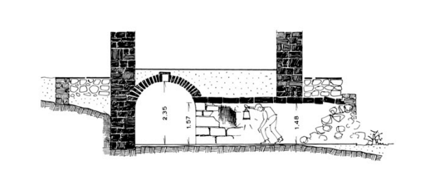
Εγκάρσια τομή 3-3 | κλίμακα 1:200
