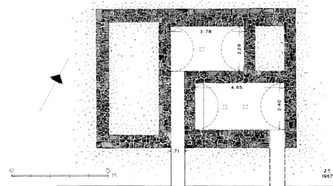
Κάτοψη κρυπτών (αναπαράσταση) | κλίμακα 1:200
