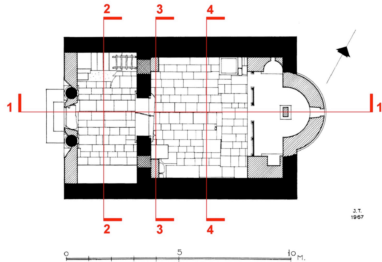
Κάτοψη ναού | κλίμακα 1:100
