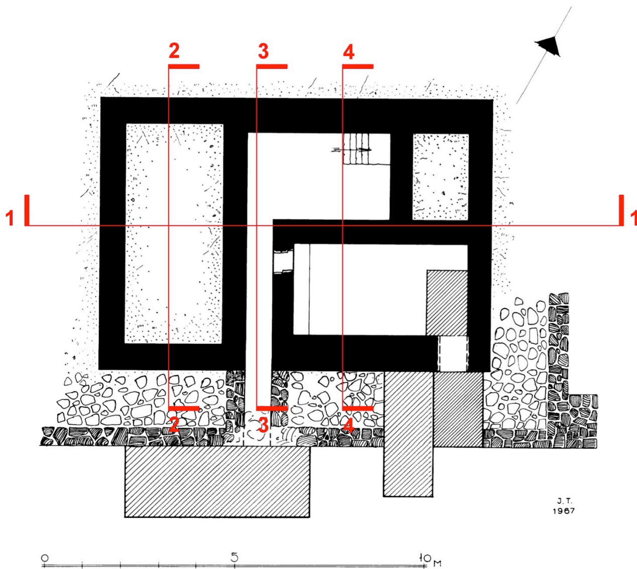
Κάτοψη κρυπτών | κλίμακα 1:100
