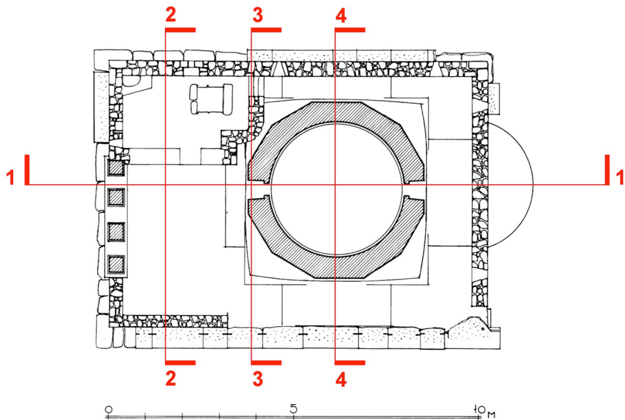
Κάτοψη στέγης | κλίμακα 1:100
