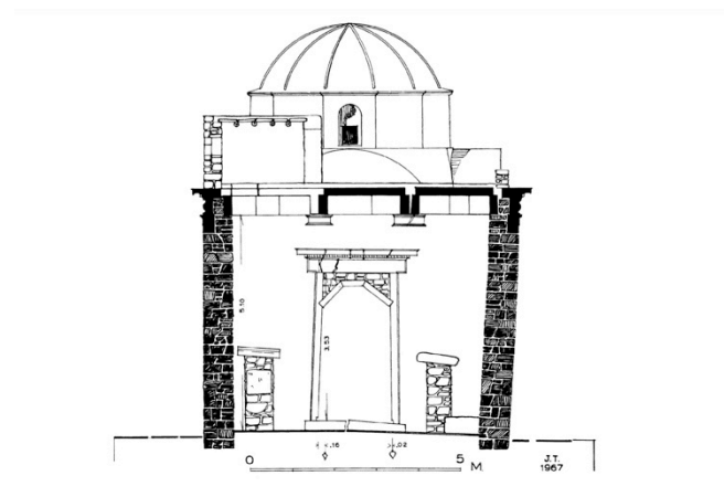
Εγκάρσια τομή 2-2 | κλίμακα 1:200
