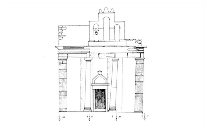
Κύρια όψη ναού | κλίμακα 1:200
