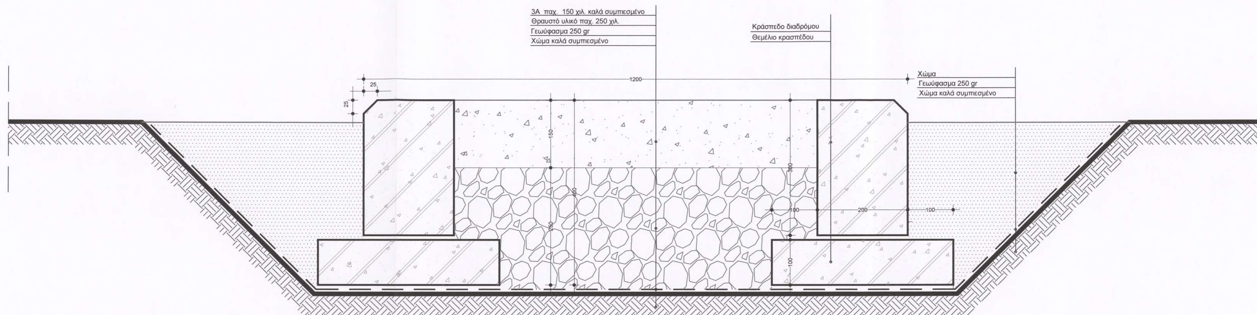
Λ.01 ΤΥΠΙΚΗ ΛΕΠΤΟΜΕΡΕΙΑ ΔΙΑΜΟΡΦΩΣΗΣ ΔΙΑΔΡΟΜΟΥ ΕΠΙΣΚΕΠΤΩΝ (οι διαστάσεις σε mm)
