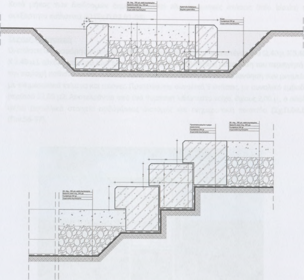
Πιν. 54 Κατασκευαστικές λεπτομέρειες διαδρόμου επισκεπτών.
