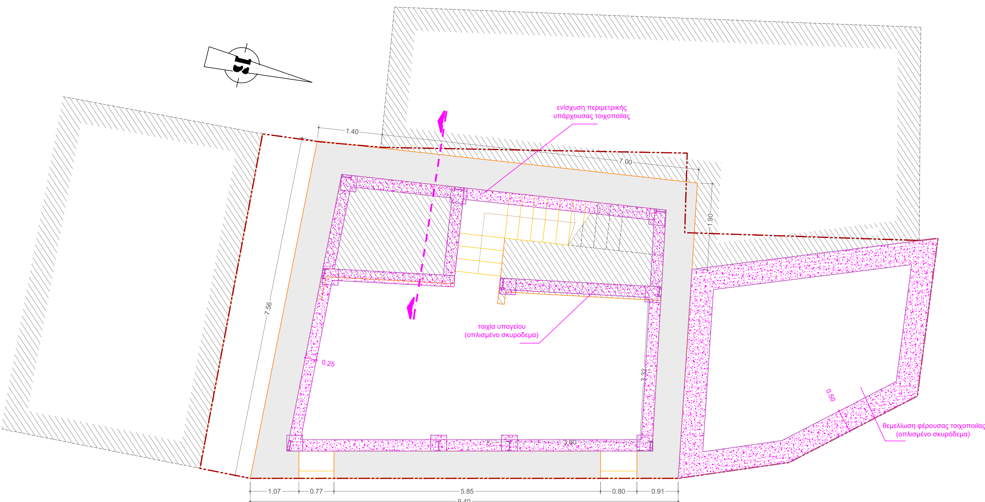
ΚΑΤΟΨΗ ΥΠΟΓΕΙΟΥ ΣΤΑΘΜΗ ΘΕΜΕΛΙΩΣΗΣ
