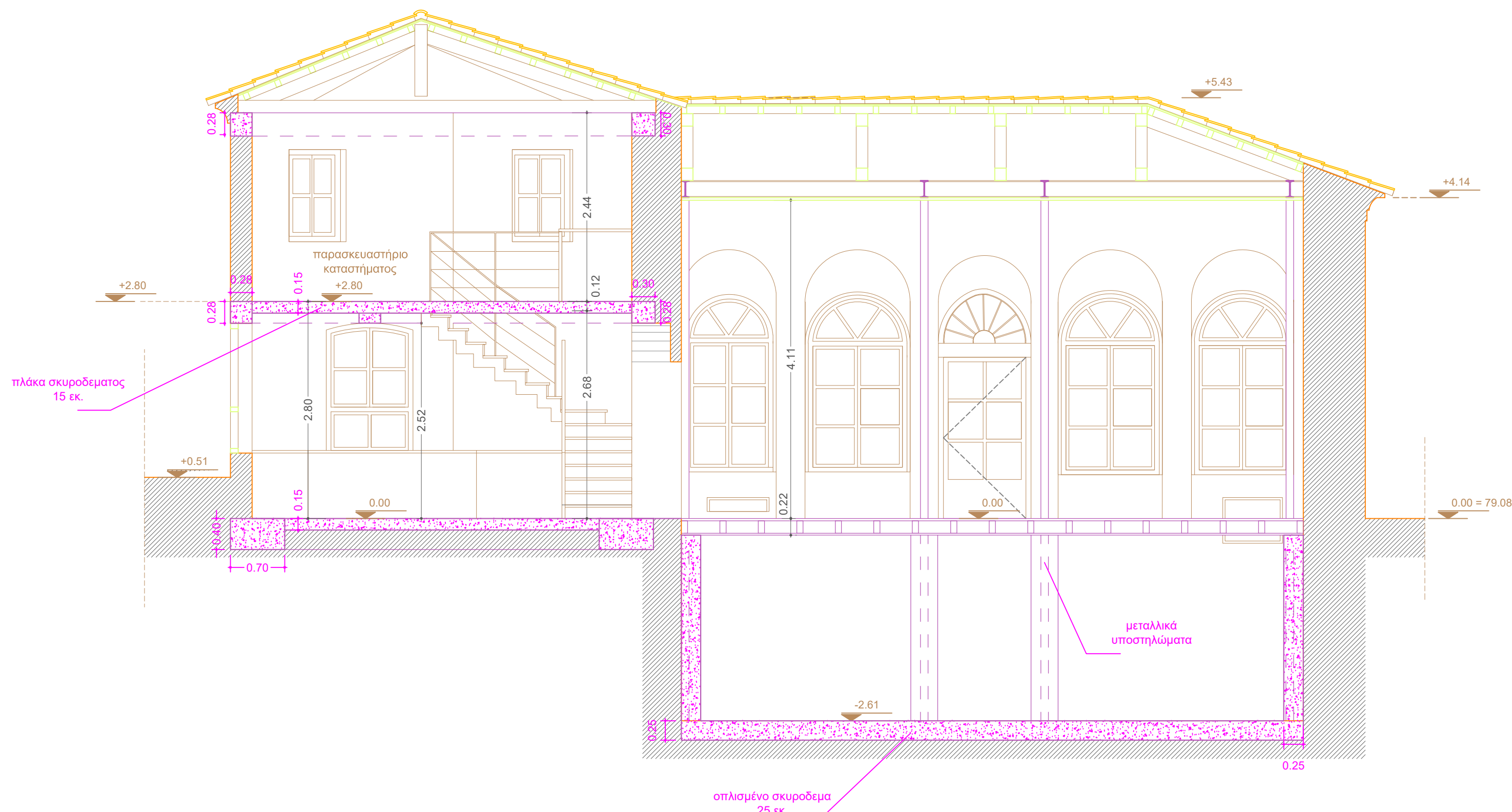
ΚΑΤΑ ΜΗΚΟΣ ΤΟΜΗ
