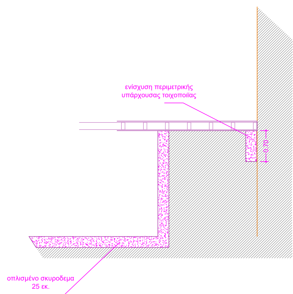
ΣΧΗΜΑΤΙΚΗ ΤΟΜΗ-ΛΕΠΤΟΜΕΡΕΙΑ
