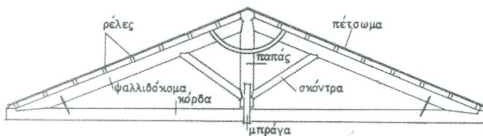
Εικ. 2. Τυπική ξύλινη στέγη στα Ιόνια νησιά και η ονοματολογία της (Ζήβας 1984, εικ. 63).
