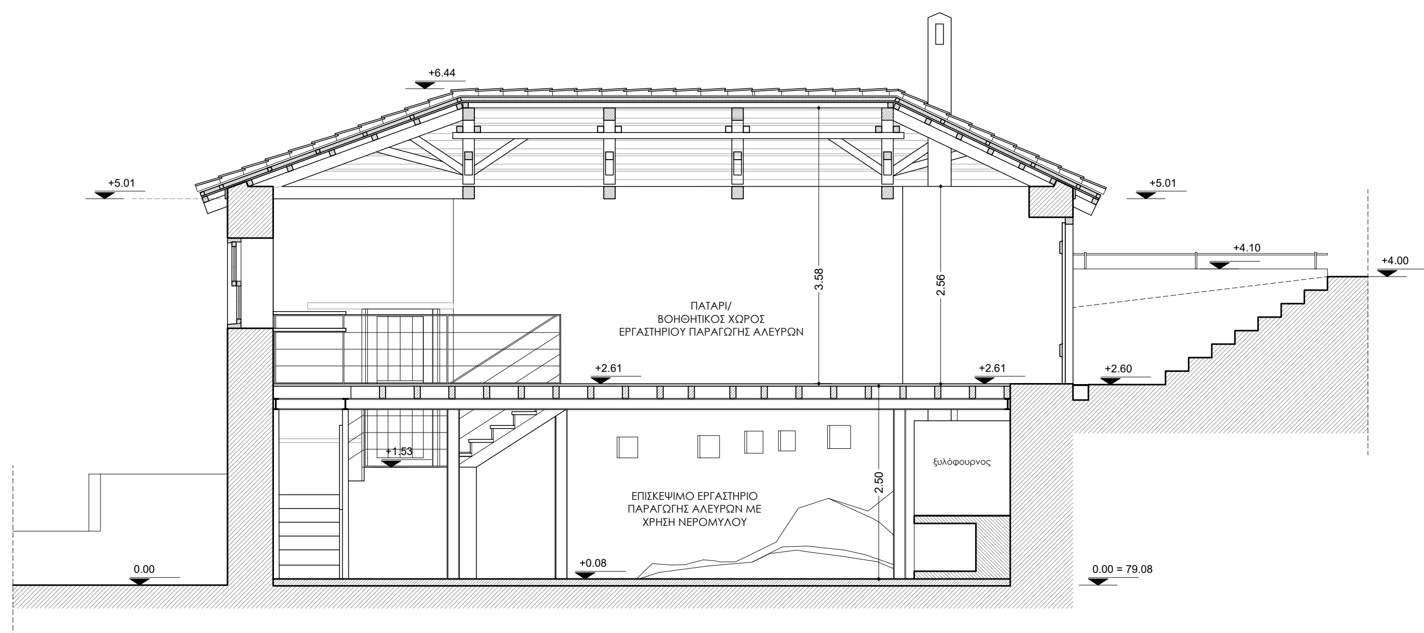
ΠΑΛΑΙΟΣ ΝΕΡΟΜΥΛΟΣ ΞΑΝΘΗΣ ΤΟΜΗ Α-Α
