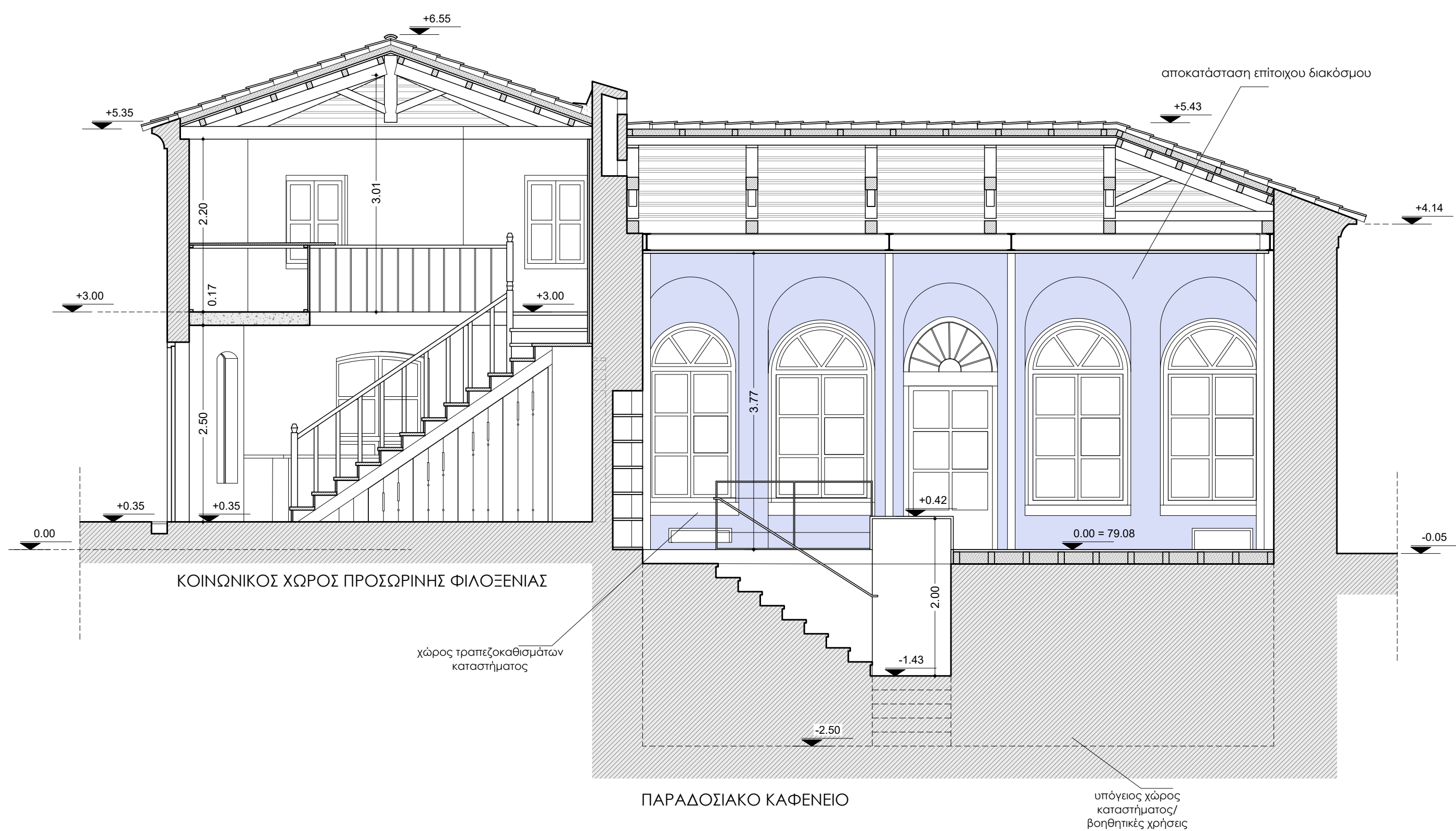
ΤΟΜΗ Γ - Γ
