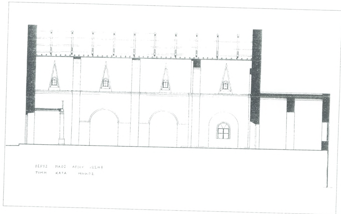
94β. Τομή κατά μήκος.
