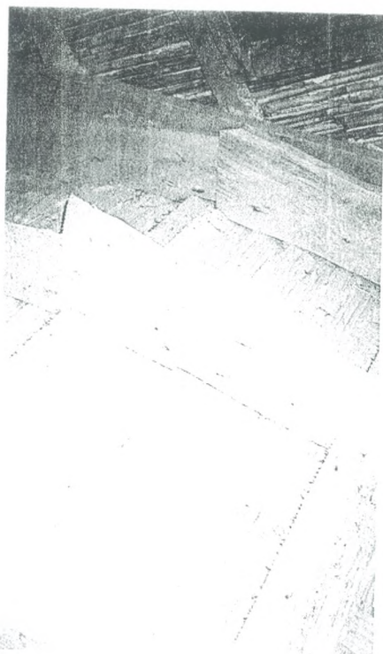
95. Λεπτομέρεια κατασκευής θόλου. Φαίνονται οι καρφωμένες μεταξύ τους ξύλινες τάβλες, τα πηχάκια που τις συγκρατούν και το καλάμωτό πλέγμα.
