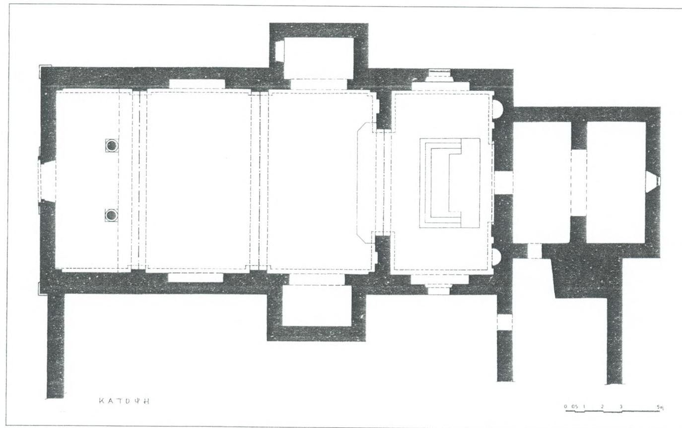
94α. Κάτοψη
