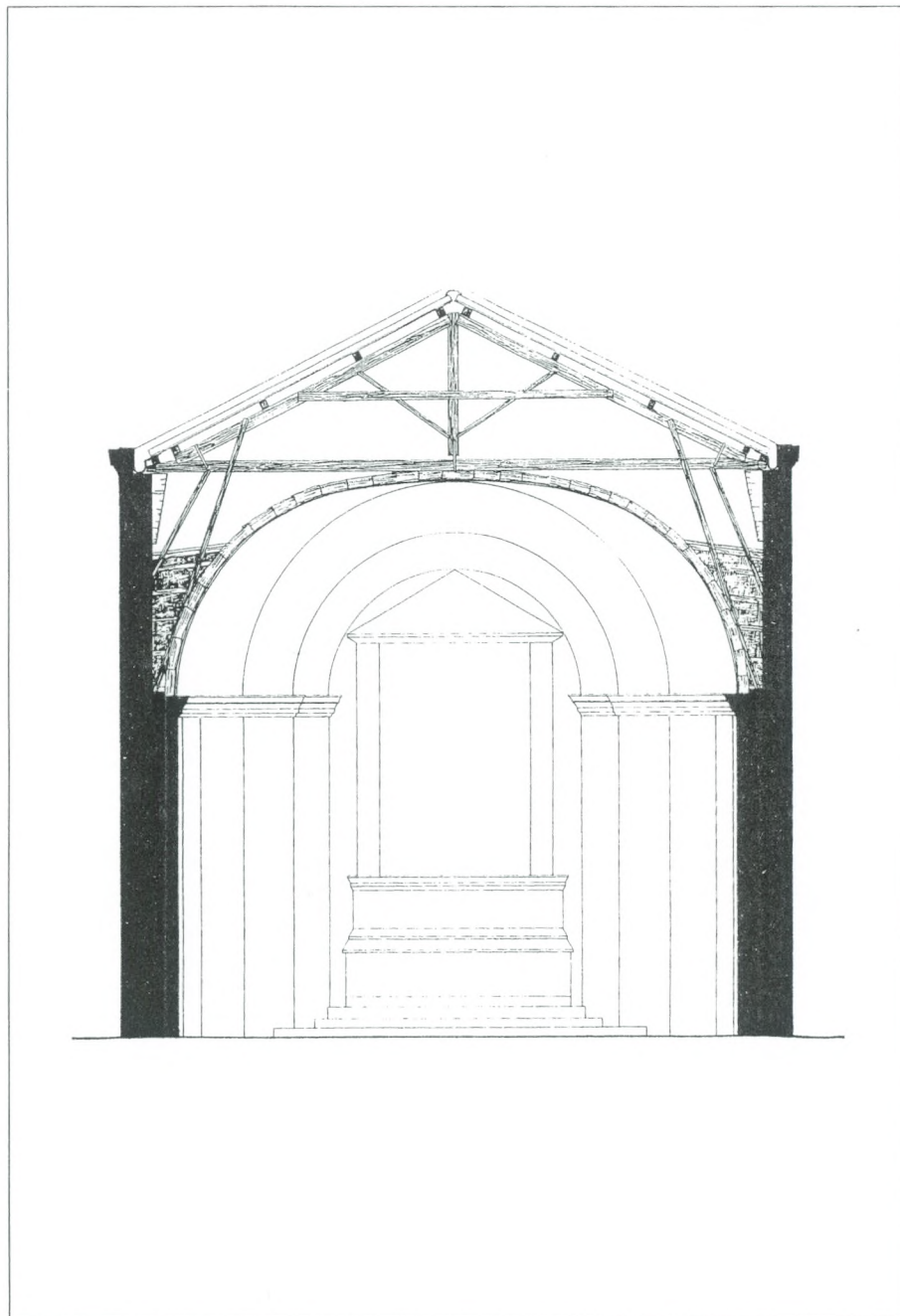
94γ. Εγκάρσια τομή.
