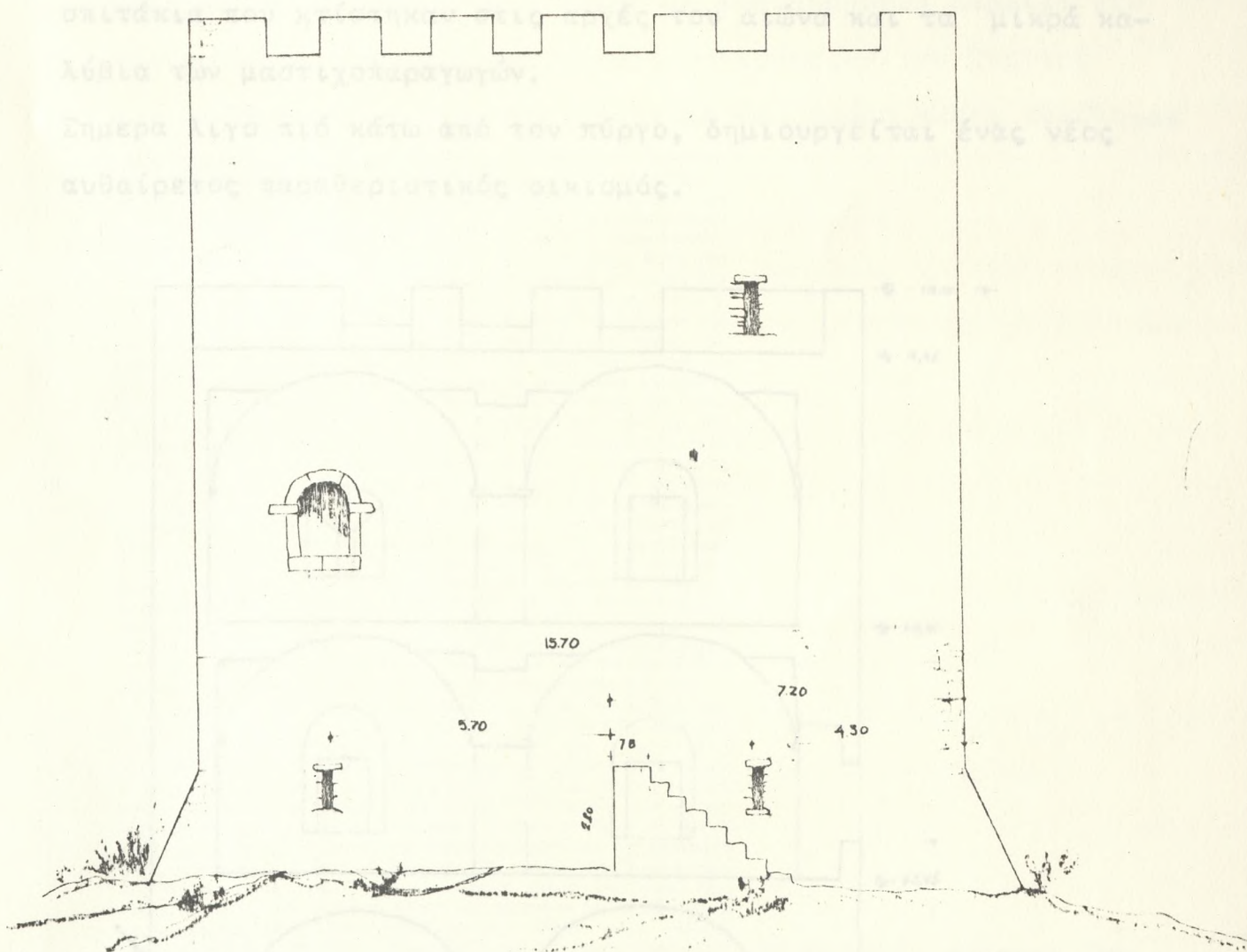
ΚΥΡΙΑ ΟΨΗ ΠΥΡΓΟΥ ΔΟΤΡΙΩΝ
