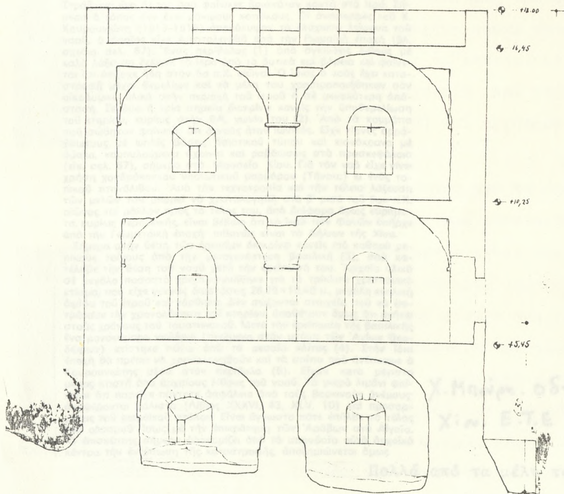
ΤΟΜΗ Α-Α ΠΥΡΓΟΥ ΔΟΤΙΕΝ
